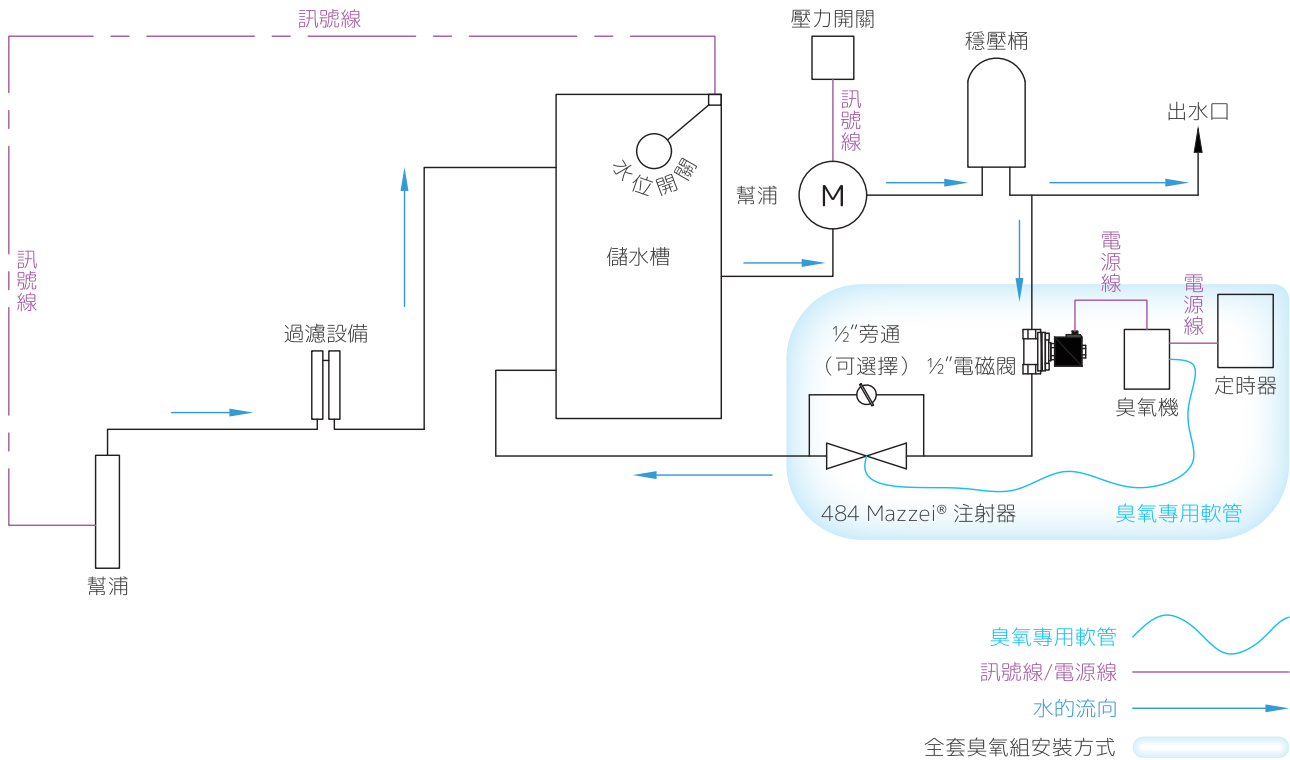
管線安裝圖 1
