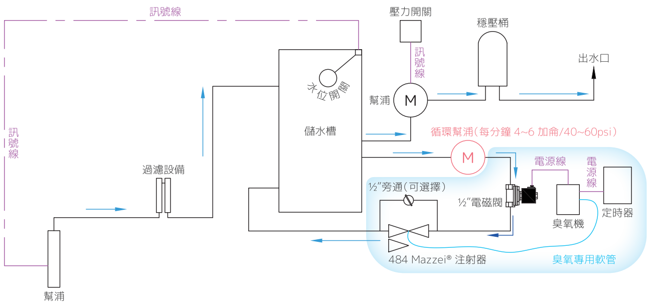
管線安裝圖 2
