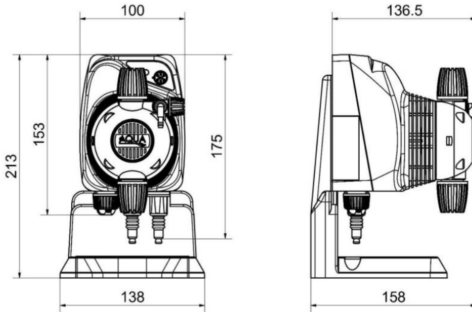
FIG. 2: SERIE "HC150" CON BASE – BASE MOUNTING
