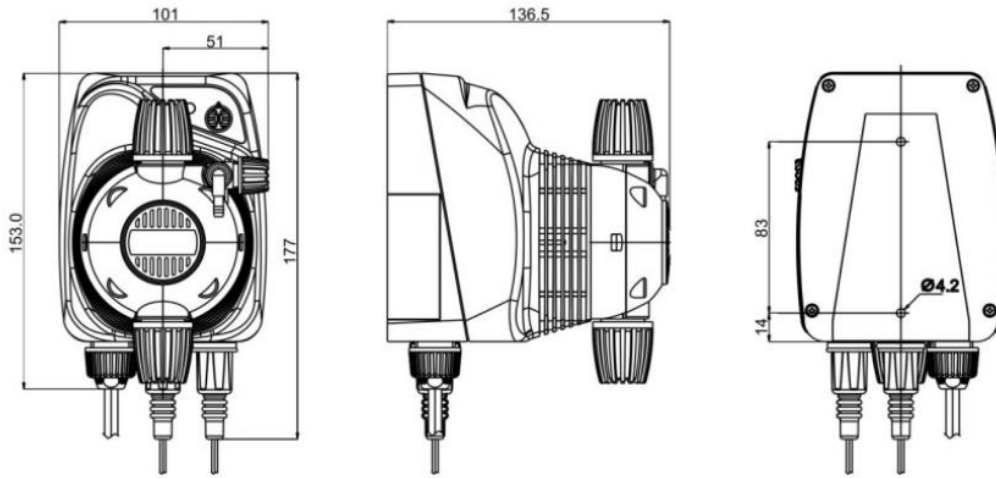
FIG. 1: SERIE "HC150" A MURO – WALL MOUNTING
